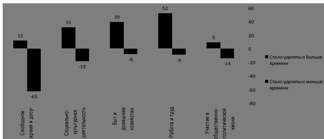
Рис. 2. Динамика сфер
